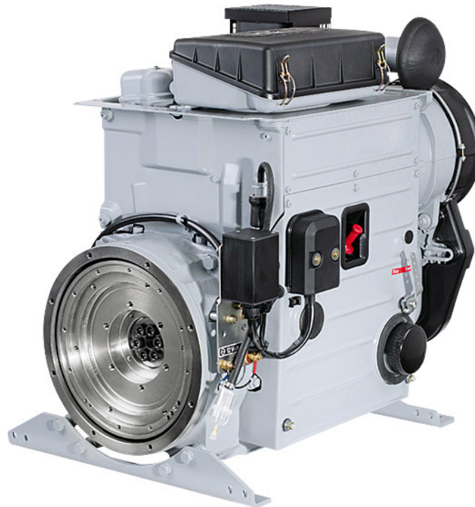
HATZ 3M41
